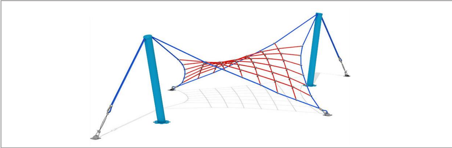
AP.1712 (Top) DIMENSIONS | 4300 X 9400 X 2500 mm
